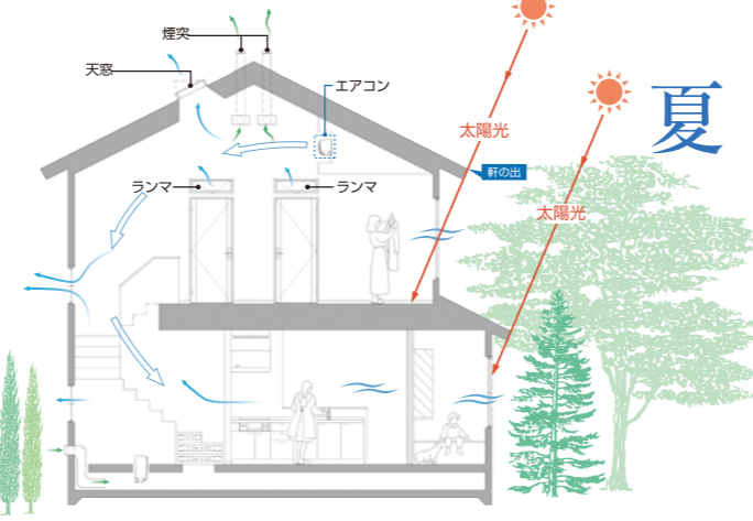
夏 は、太陽の陽差しを上手に遮光・遮熱し、室内の熱気は高窓（天窓等）から逃がす工夫で、全館快適。
