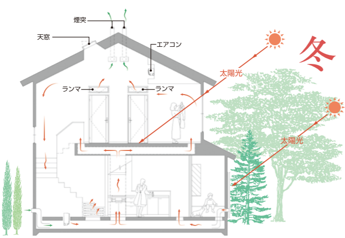
冬 は、太陽の陽差しを上手に室内に取り込んで、蓄熱した熱を暖房の補助として使用します。床下暖房で全館快適。
